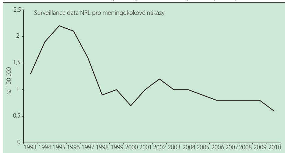
Graf 1. Nemocnost invazivním meningokokovým onemocněním, Česká republika, 1993–2010
